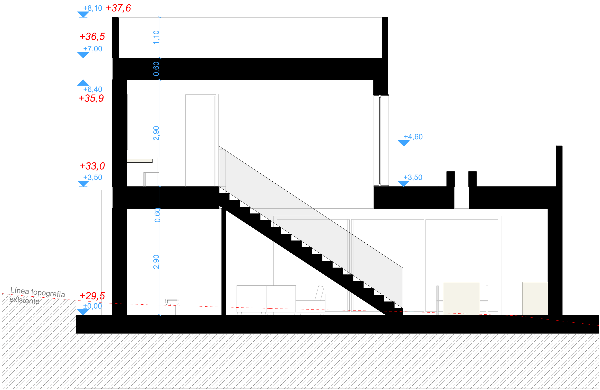
A-T Sección Transversal 1:50
