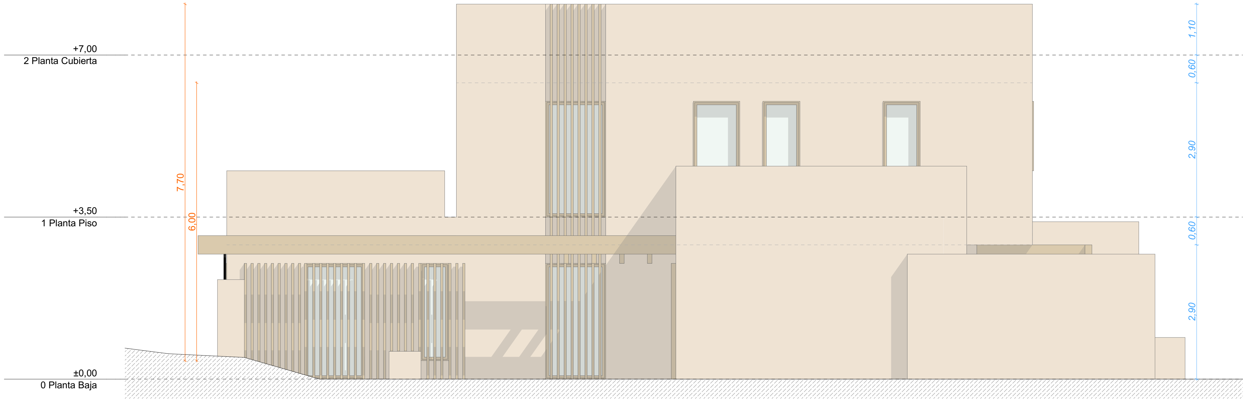
A - E Alzado 1:50
