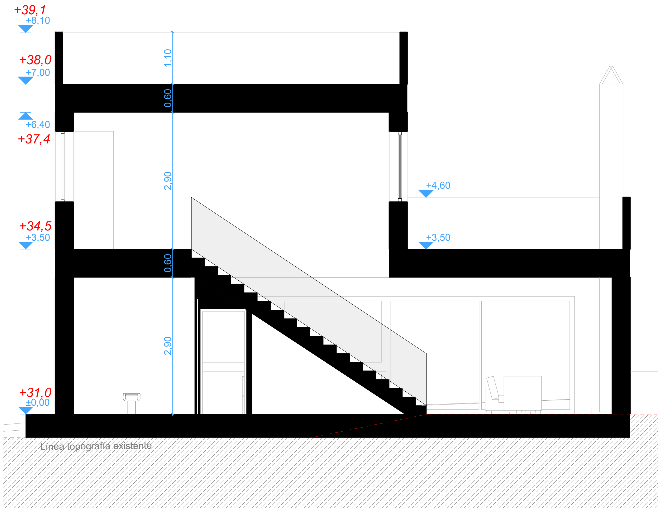
B-T Sección Transversal 1:50
