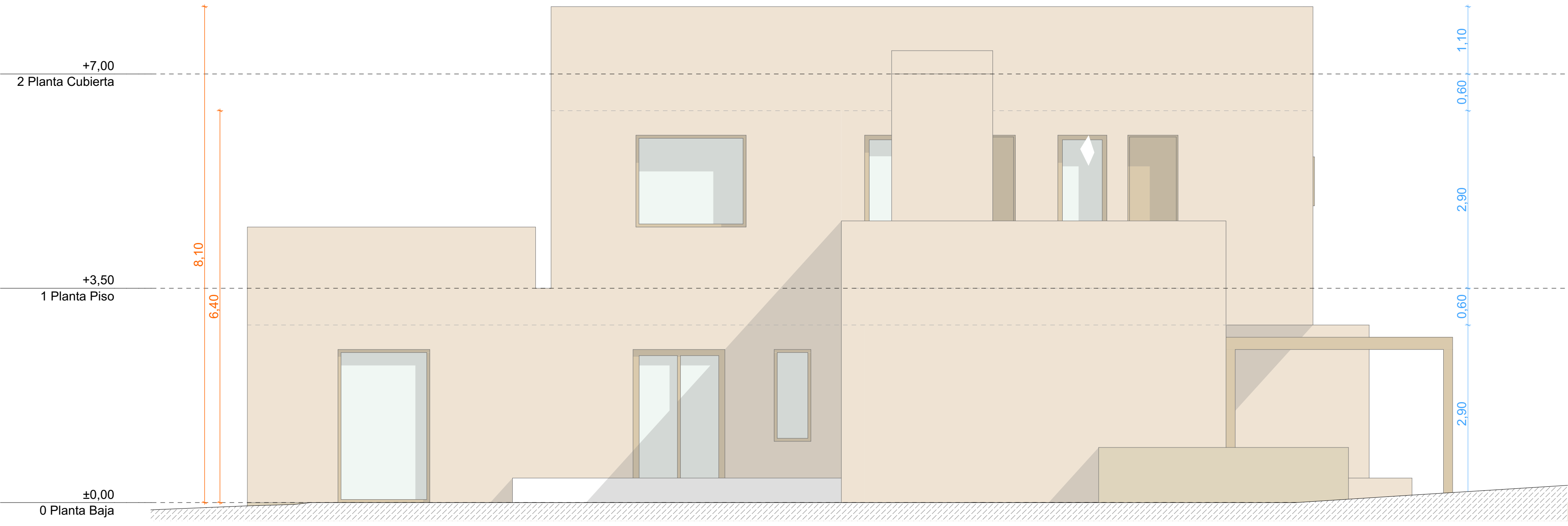
B - O Alzado 1:50
