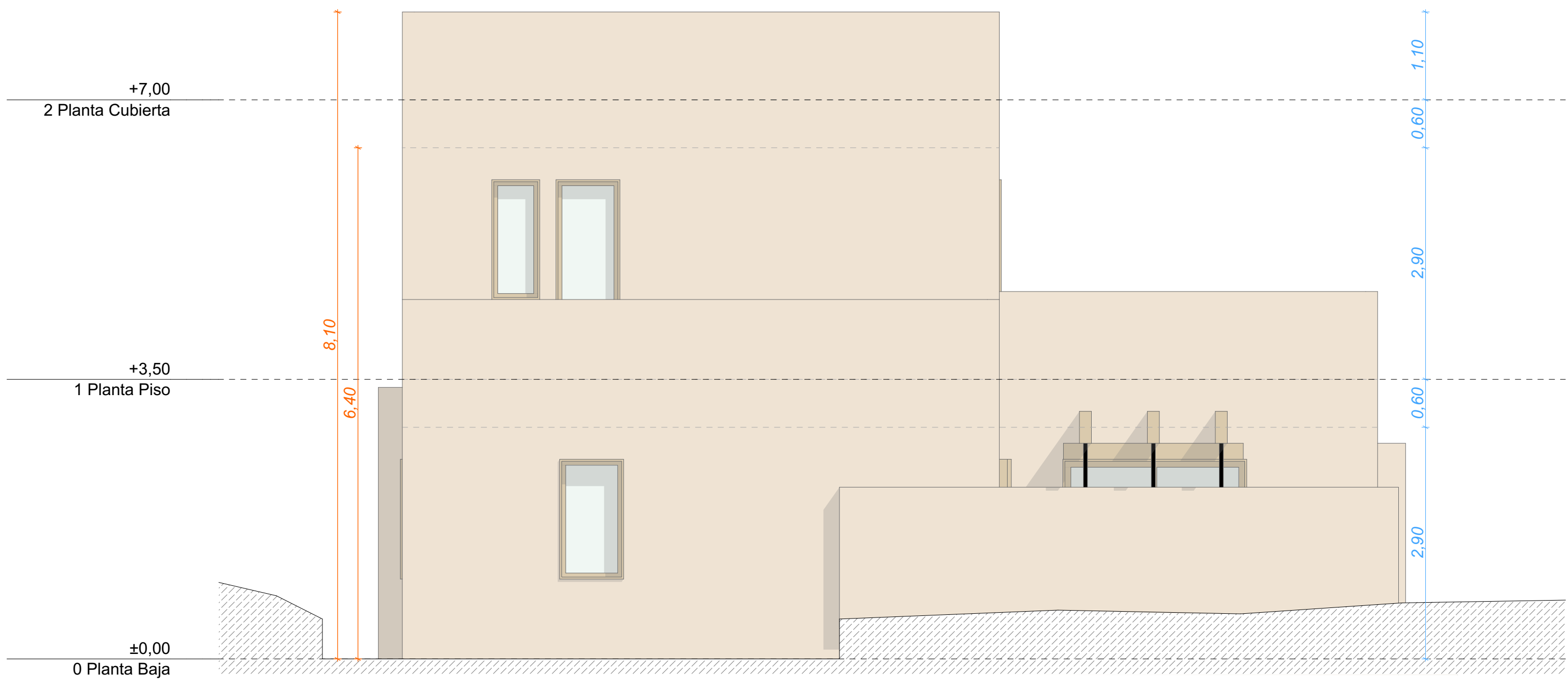
A - S Alzado 1:50
