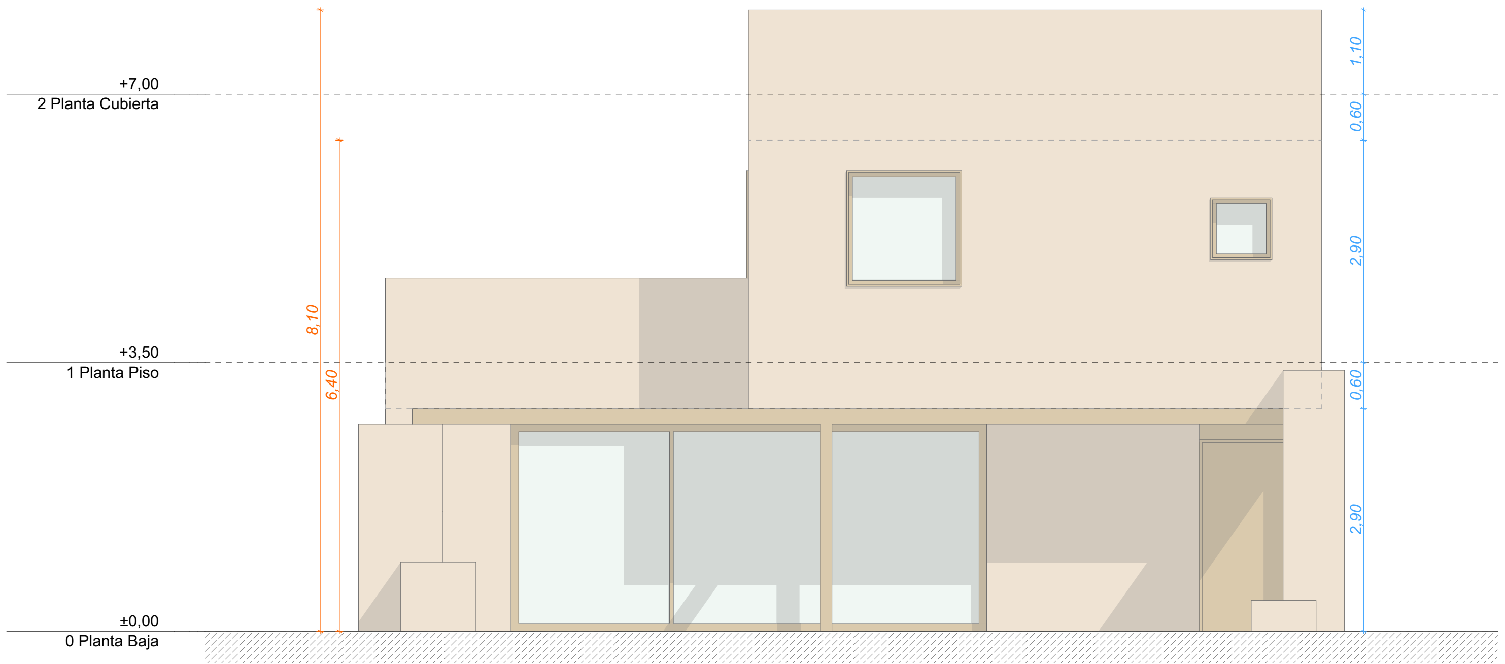
A - N Alzado 1:50
