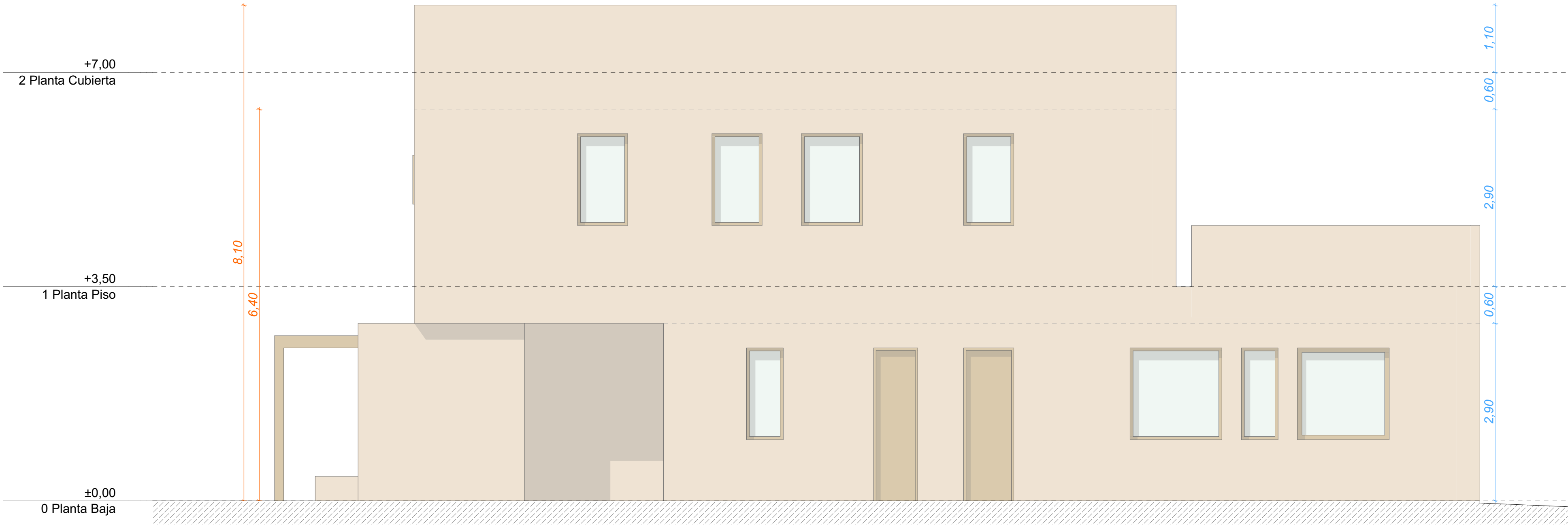
B - E Alzado 1:50
