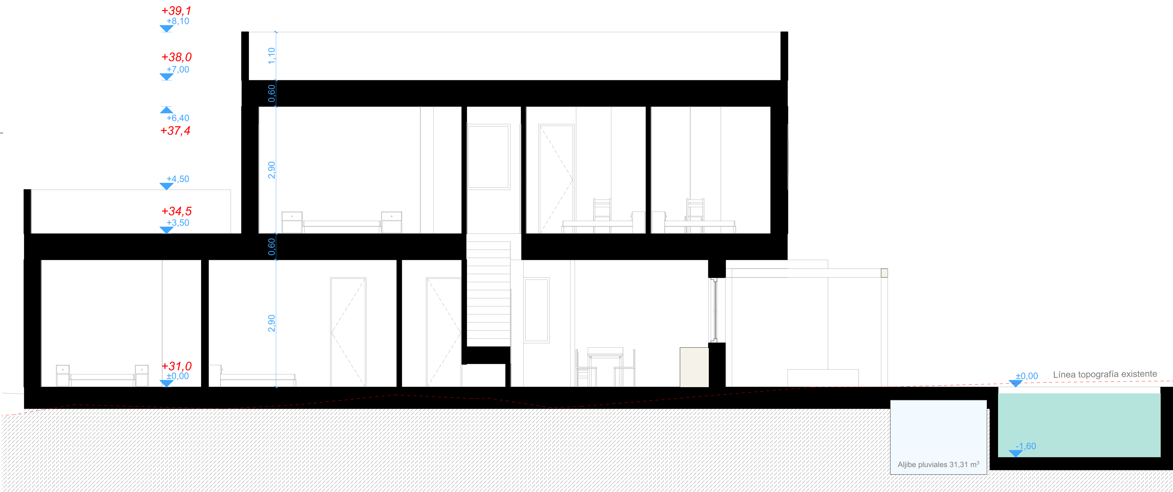
B-L Sección longitudinal 1:50
